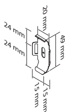
Modell XL-20 Clipsbeslag
