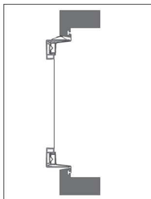
Typ 3 - ex. fönsterram i plast/trä.
