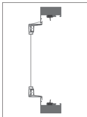
Typ 5 - ex. fönsterram i alu.
