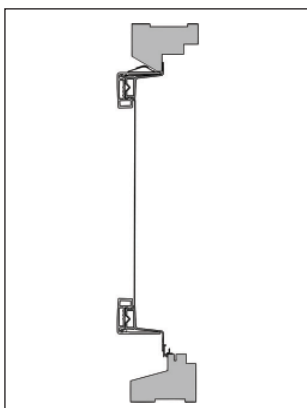
Typ 4 - ex. fönsterram i trä.
